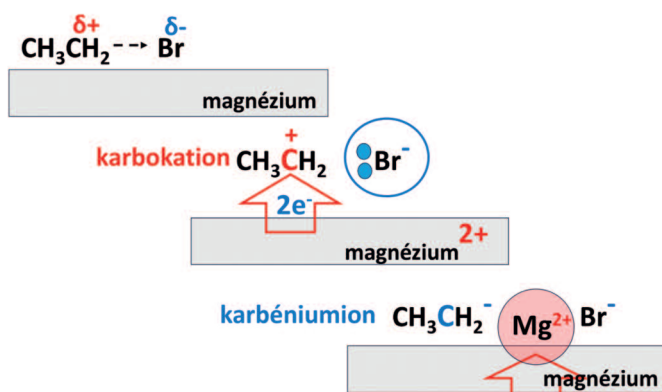
4. ábra. A magnézium felületén megkötődő etil-bromid elektrofil centruma vonzza a fém delokalizált elektronjait. A letaszított „bróm” a kötő elektronpárral együtt bromidion formájában távozik. Az elektronhiány következtében az elektrofil szénatom – rövid élettartamú – karbokationná alakul. Az oxidációt előidéző centrum a két elektron átvétele által redukálódik, és karbénium-ionként a magnéziumion másik ellenionjává válik
