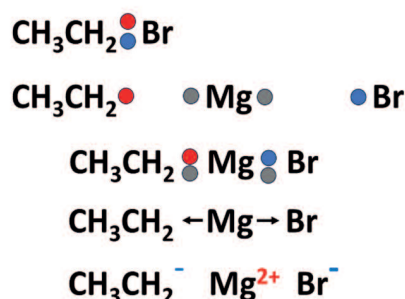
3. ábra. A magnéziumatom beékelődése kovalens jellegű kötés kialakulásával. A magnéziumatom egy-egy elektronja kötésként alakít ki a szén-brom kötés szétválasztott kötő elektronpárjának egy-egy elektronjával, majd a kötések az elektronegativitás-különbségnek megfelelően polarizálódnak
