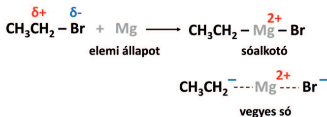
2. ábra. Az elemi állapotú „magnézium” vegyes sót alkotva beépül a szerves és a szerves anion közé
