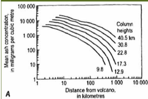
5. ábra: A Csendes-óceán parti Mt. St. Helen kitörési oszlopának szétterjedése
