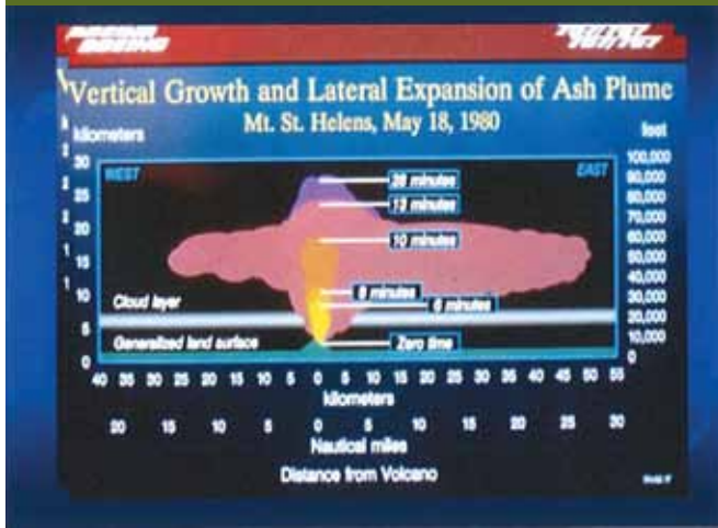
5. ábra: A Csendes-óceán parti Mt. St. Helen kitörési oszlopának szétterjedése
