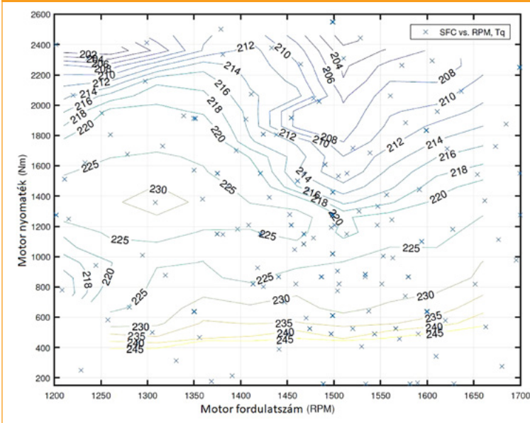
6. ábra: Egy hajómotor fajlagos tüzelőanyag-fogyasztás térképével - fuel map (forrás: [12])
