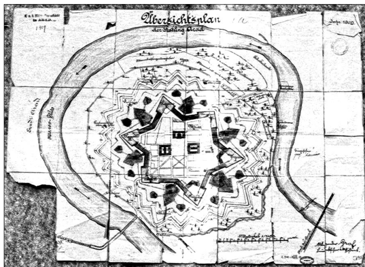
Az új aradi vár tervrajza
