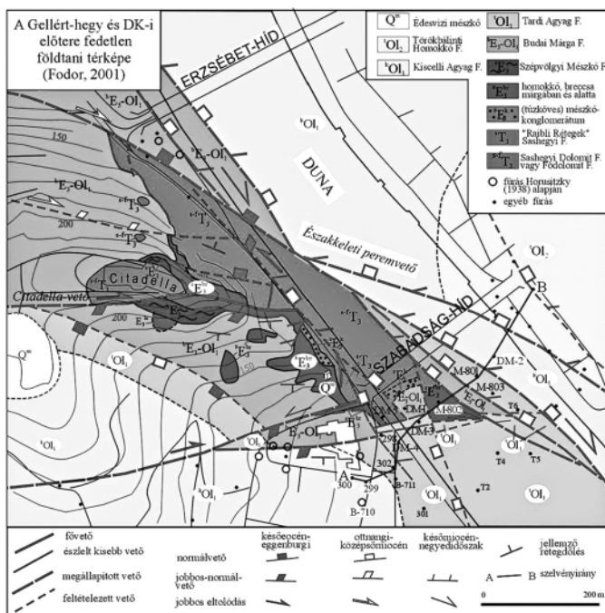
A Gellért-hegy és DK-i előterének fedetlen földtani térképe (Fodor 2001)
