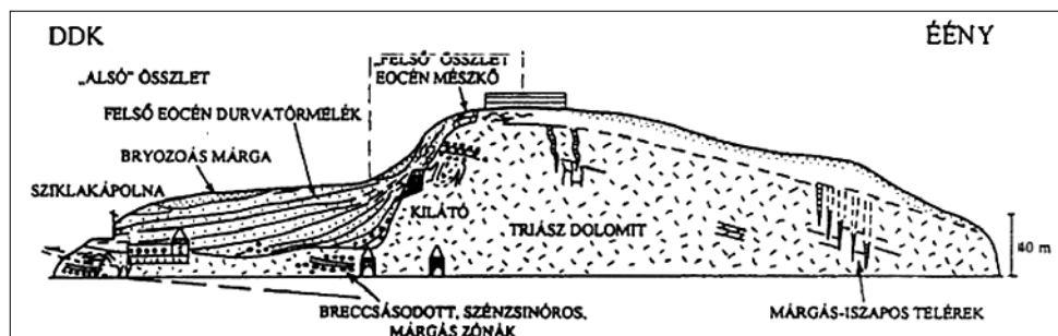
A Gellért-hegy keleti falának földtani metszete (Magyari 1996, in Korpás et al. 2002)
