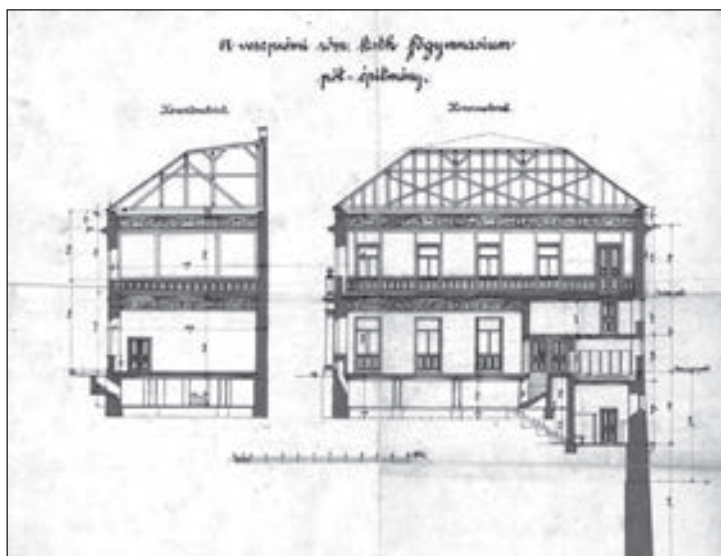
26. A rajzterem és díszterem épületének (gimnázium D-i szárny) tervrajzai, metszetek. Schmahl Henrik építész, 1901. 68
