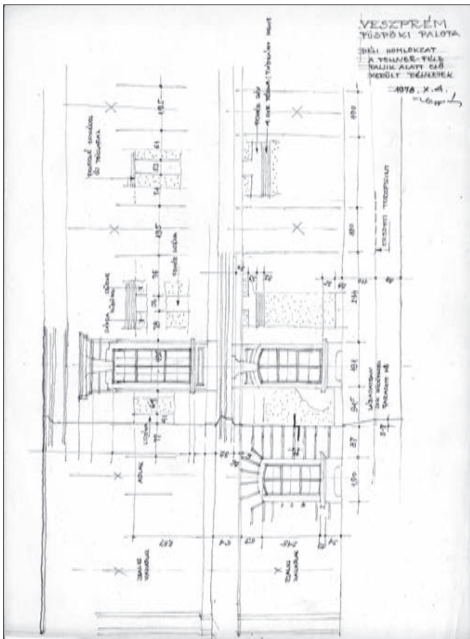
A déli homlokzat kutatási rajza (Rajz: Koppány Tibor)
