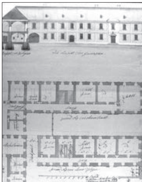
14. Strakovich Sebestyén kőművesmester terve a gimnázium bővítésére, 1843 (nem valósult meg). 57
