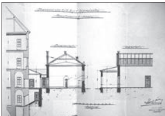
23. Tervrajz a tornaterem felépítésére a gimnázium épületéhez csatlakoztatva, 1899 (nem valósult meg), metszetek. 65
