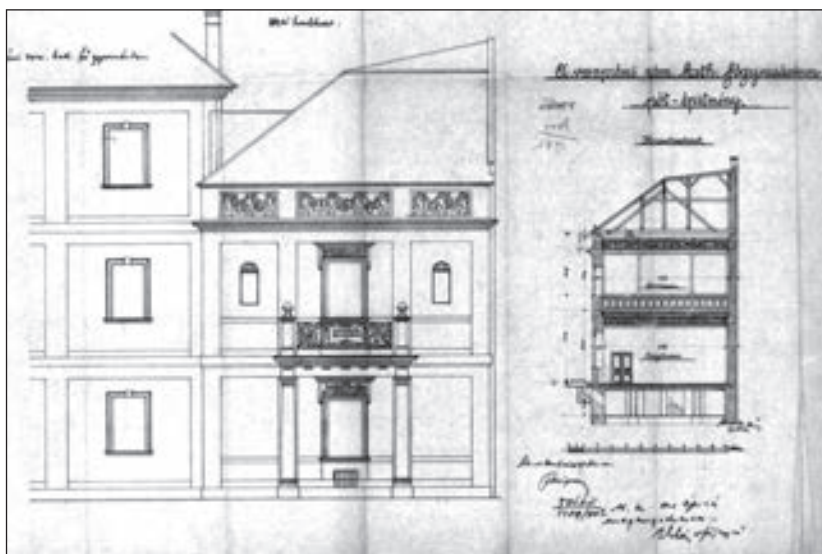
25. A rajzterem és díszterem épületének (gimnázium D-i szárny) tervrajzai, Ny-i homlokzat és keresztmetszet. Schmahl Henrik építész, 1901. 67
