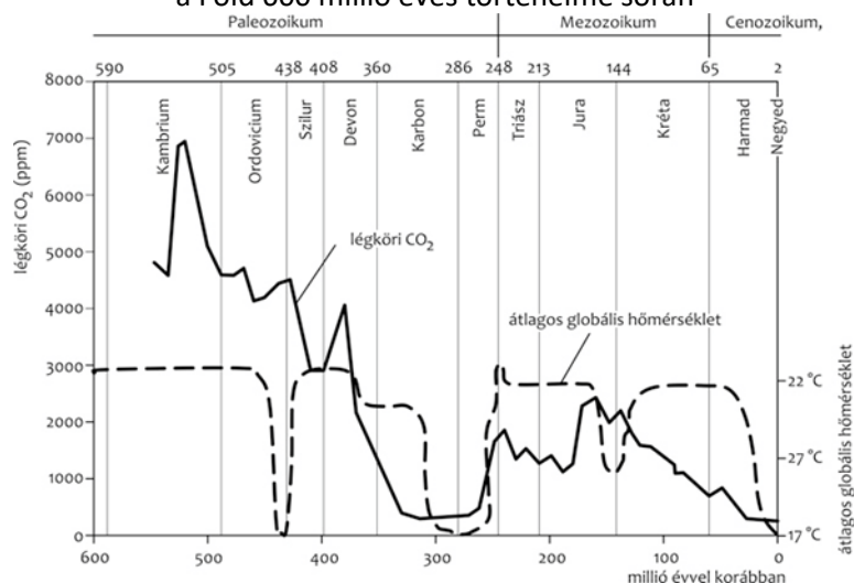
Az átlagos CO 2 -koncentráció és a globális hőmérséklet alakulása a Föld 600 millió éves történelme során
