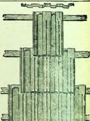
ZSOMBOLYAI gyártmány. Szab. biztonsági átfedő cserep 272 sz.
