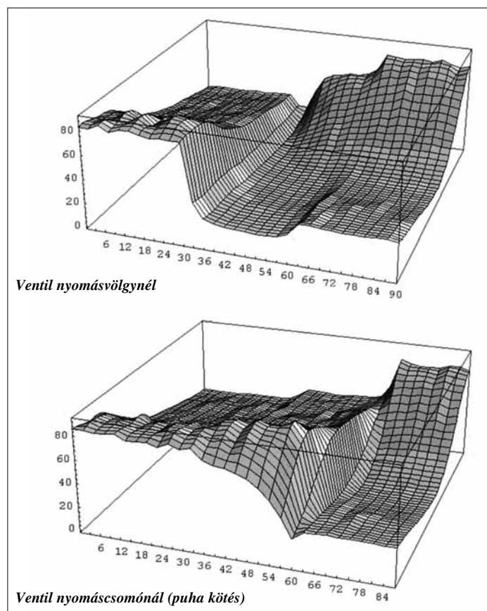
8. ábra: impedancia lefutása egy egészhangos kötés alatt
