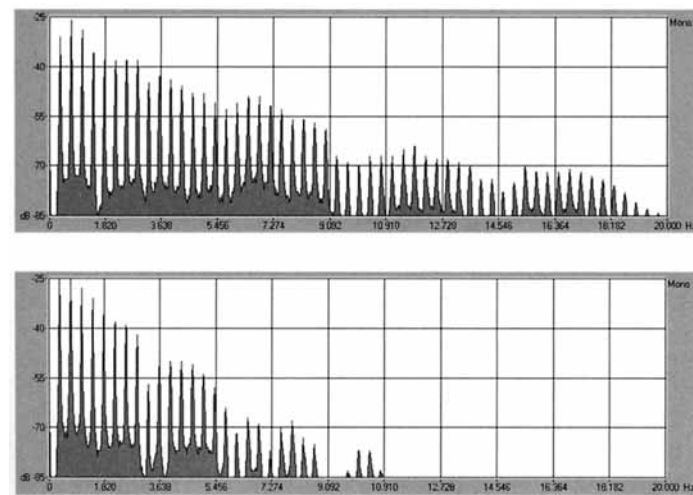
9. ábra: egy fortissimóban játszott leírt c" hangspektruma. Főnt bécsi kürtől, lent: egy távol menzúrált triplakürt magas f-kürt részén.
