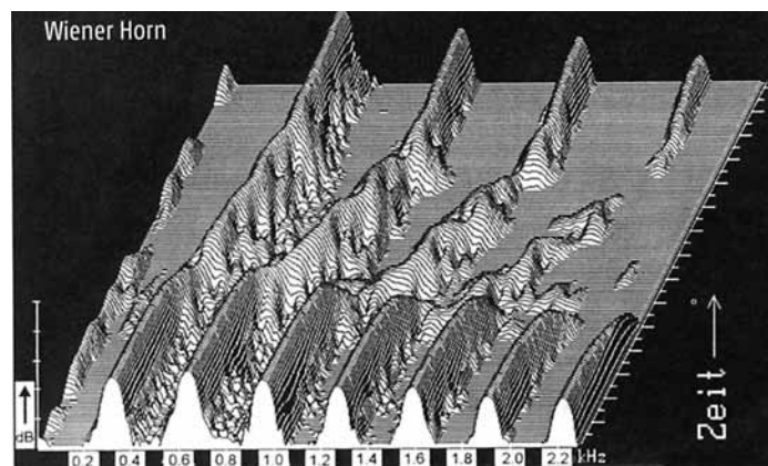
6. ábra: egy kötés három dimenziós ábrázolása bécsi kürtön. Időselet: 1 mp
