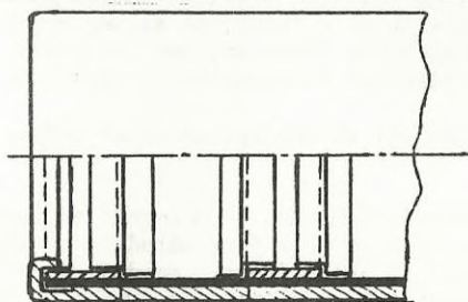
1. ábra. A cső félnézet-félmetszetben ábrázolva
