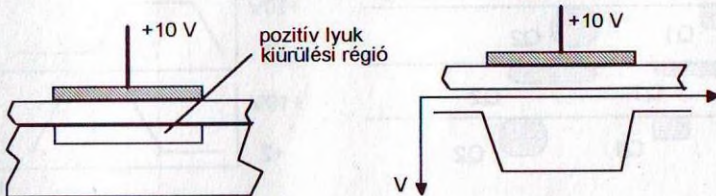
2. ábra. A pozitív lyuk kiürülési régió elhelyezkedése a félvezető alaprétegben és a feszültség „eloszlása” az elektróda alatt
