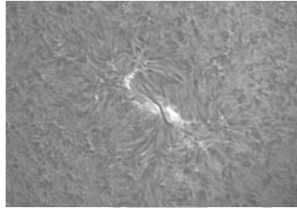
Áldott Gábor felvétele a 12759-es régióról 2020. április 6-án 15:20 UT-kor készült, 80/1200-as Zeiss AS refraktorral, ASI-120MM-S kamerával (PST H \alpha szűrő). A csoportot fotoszférában már nem lehetett megfigyelni, azonban a kromoszférában még napokig jól láthatóan volt a terület
