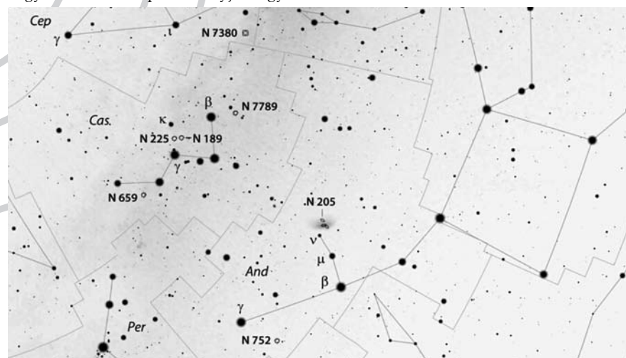
Néhány a Caroline Herschel által felfedezett objektumok közül (Stellarium)
