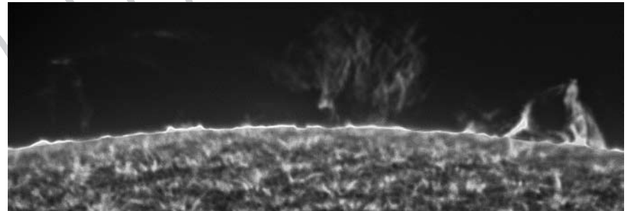
Horváth Attila Róbert részletgazdag felvétele a kromoszféráról 2020. augusztus 31-én készült 127/1200-as refraktoral, Luns 50LS hidrogén-alfa szűrővel, ASI 178MM kamerával, 3000 mm-es eredő fókusszal. A felvételen gyönyörű protuberanciákat figyelhetünk meg és a kromoszféra felületén a szpikulák is feltűnnek
