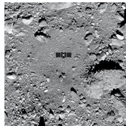
Az Osiris-REX szonda „Csalogány” nevű kijelölt leszállóhelye a Benu felszínén (NASA)
