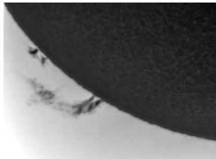
Szabó Szabolcs Zsolt felvétele 2020. február 11-én 15:57 UT-kor készült Lunt 60/500-as naptávcsővel (2x nyújtás, ZWO ASI 178 MC kamera) a nyugati peremen látható aktív, de számozatlan területéről, ahol egy hatalmas hurokprotuberanciát lehetett megfigyelni. „Óriási protuberanciahurok volt látható a délutáni órákban. A naptávcsőben percről percre változott a mozgása. Nagyjából 2–3x-os Jupiter-átmérőnyire távolodott el a kromoszférától!”
