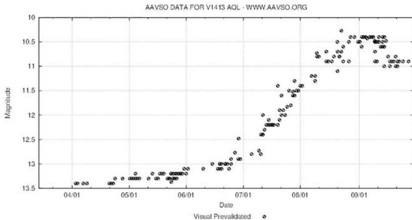
A V1413 Aql fényességváltozásai 2020 áprilisa és szeptembere között (aavso.org)
