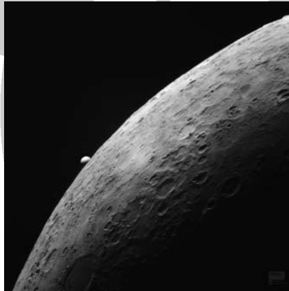
A fedés előtti pillanatban, 10:10 UT-kor készült Fényes Lóránd felvétele 160/1308 GPU APO triplet, iOptron iEQ45-mod, ZWO 533MM Pro, Astronomik ProPlanet IR Pro 742 szűrő
