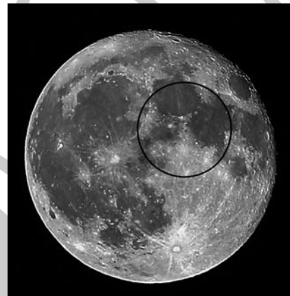
A 11 mm-es Nagler-okulár hozzávetőleges látómezeje a Holdon, 250/5000-es Cassegraintávcsővel, 451×-es nagyítással
