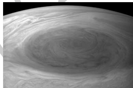
A NASA Juno-űrszondája által készített közelkép a Nagy Vörös Fotról. A felhőzet fölé mintegy 8 kilométerrel kiemelkedő struktúra a környezeténél erőteljesebben kitett az intenzív ultraibolya sugárzásnak (NASA/JPL-Caltech/Björn Jónsson)
