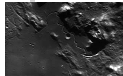
Egy számomra nagyon emlékezetes fotó a Hadley-rianásról 2015. január 28-án 18:32 UT-kor, a 250/5000-es Cassegrainnel, 10 m effektív fókusszal, QHY 5II L színes kamerával. Rendkívül ritkán kell fókusznyújtót használnom
