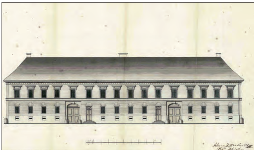
Mayerffy Xavér Ferenc serfőzdjének homlokzati terve. Zitterbarth János, 1815
