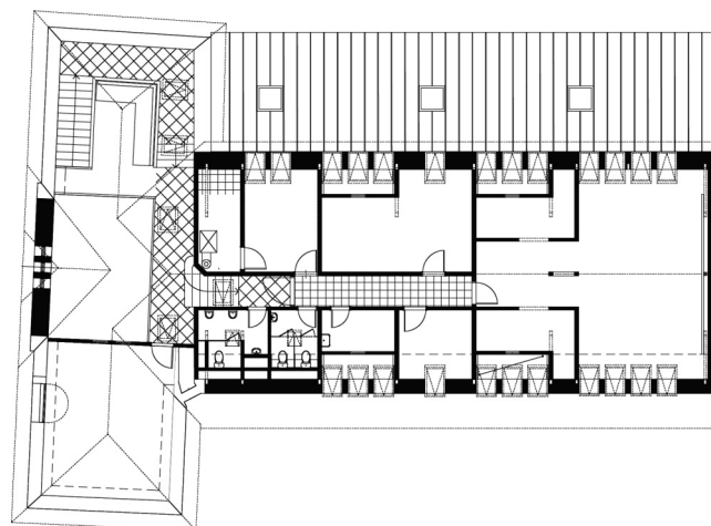
A művelődési ház tetőtérének terve
