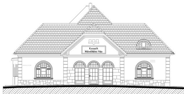
A művelődési ház tervezett homlokzati képe
