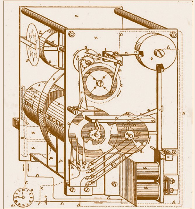
Kleiszner villamos óranaptárának rajza a párizsi La Lumière Électrique 1889. március 2-i számában
