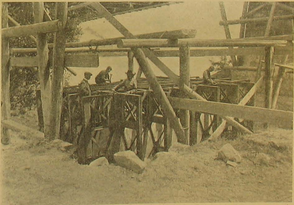
A budai hídfő caissonjának szerelése.
