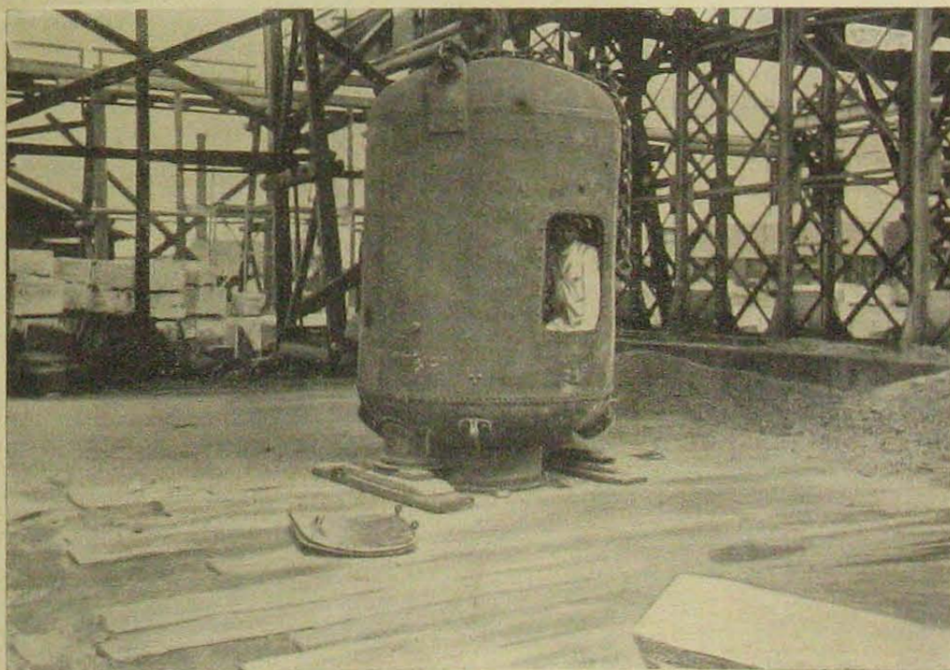
Egy caisson légszilipje.
