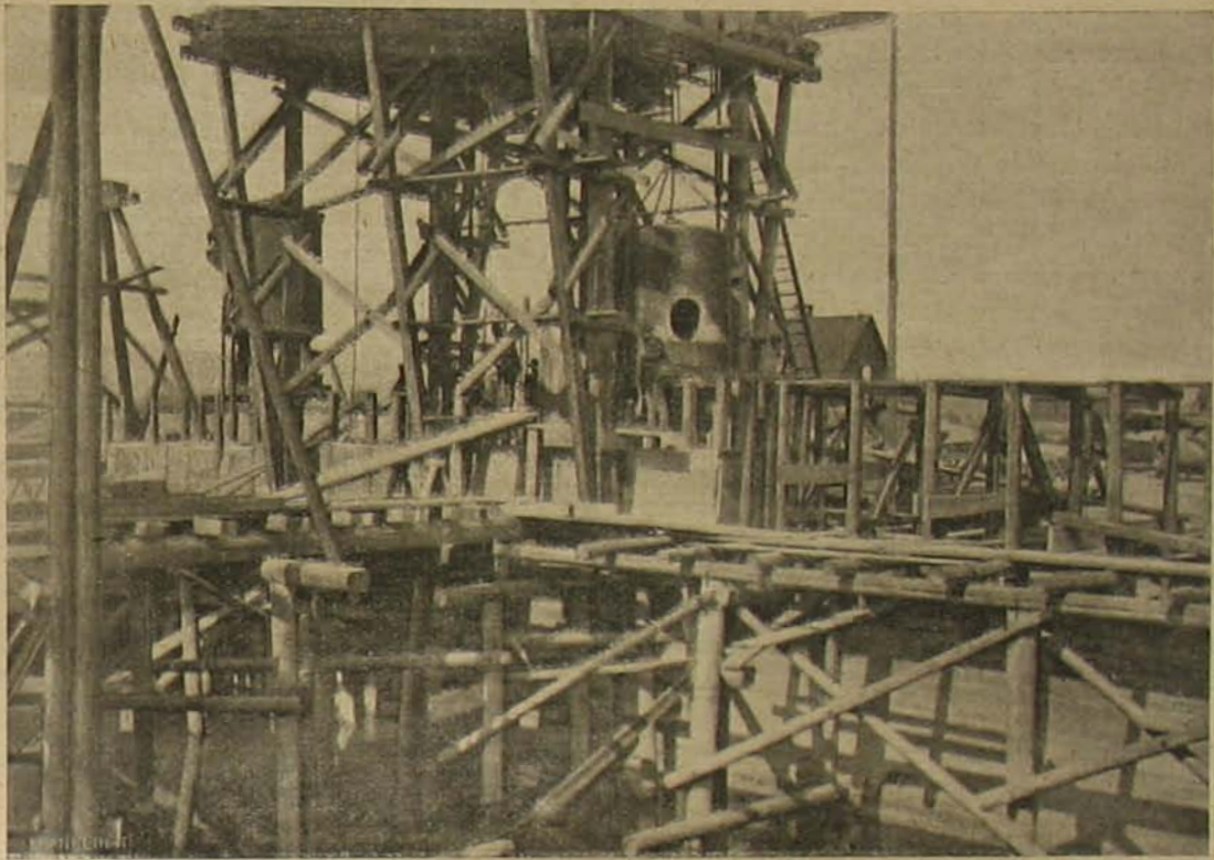
Súlyesztésre előkészített caissonok.
