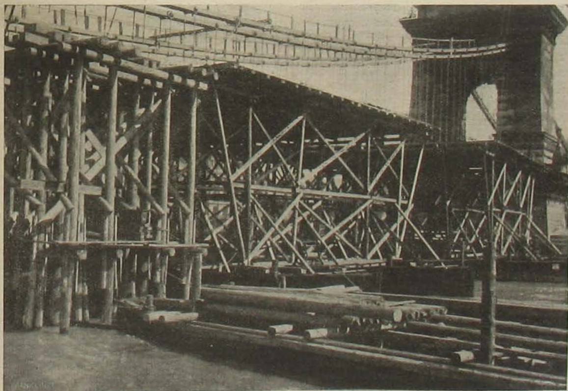
Morev és úszó állványokról szorítják le a régi láncokat.
