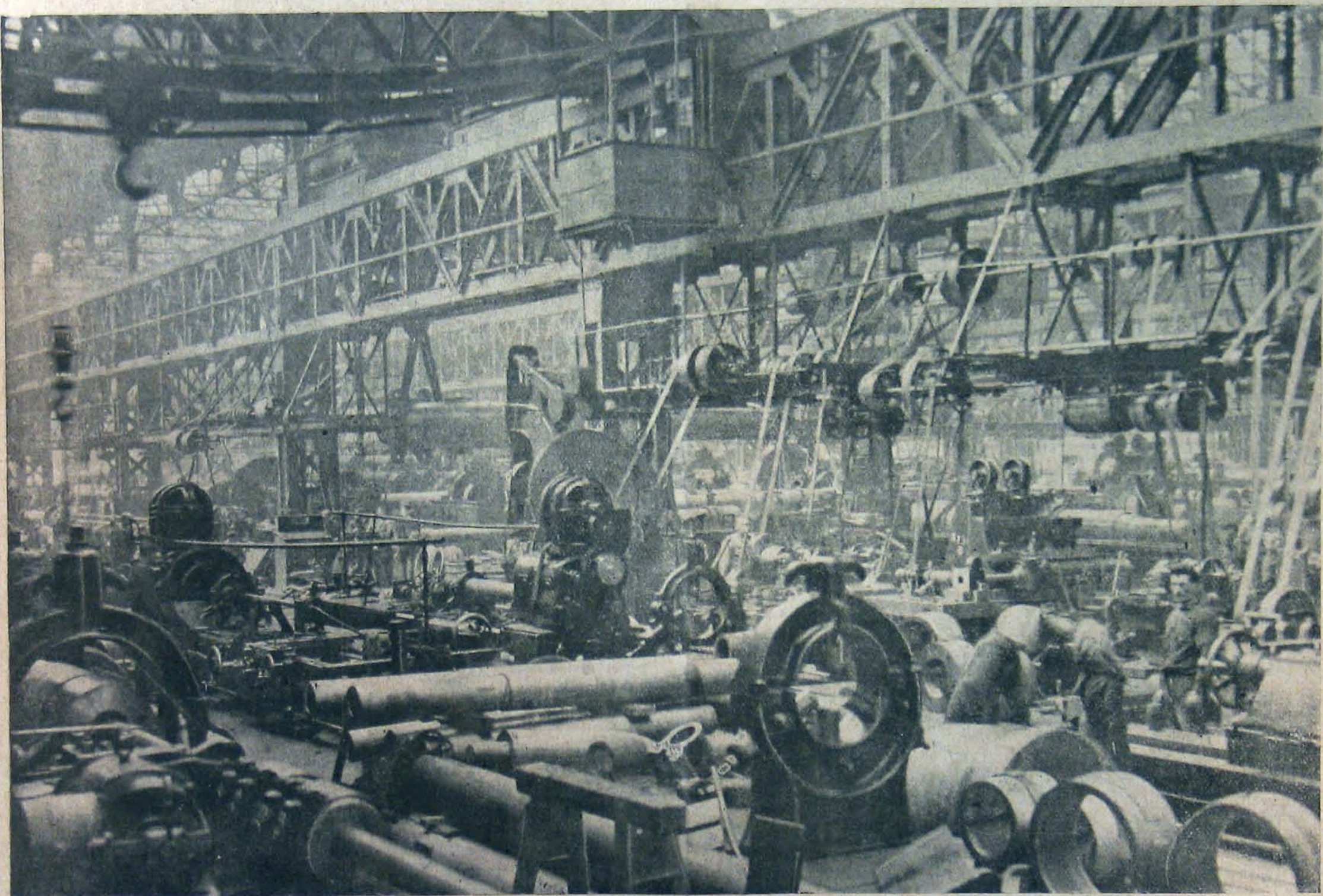
Ágyugyártás a Skodagyárban. — Agyuesztergályozás.
