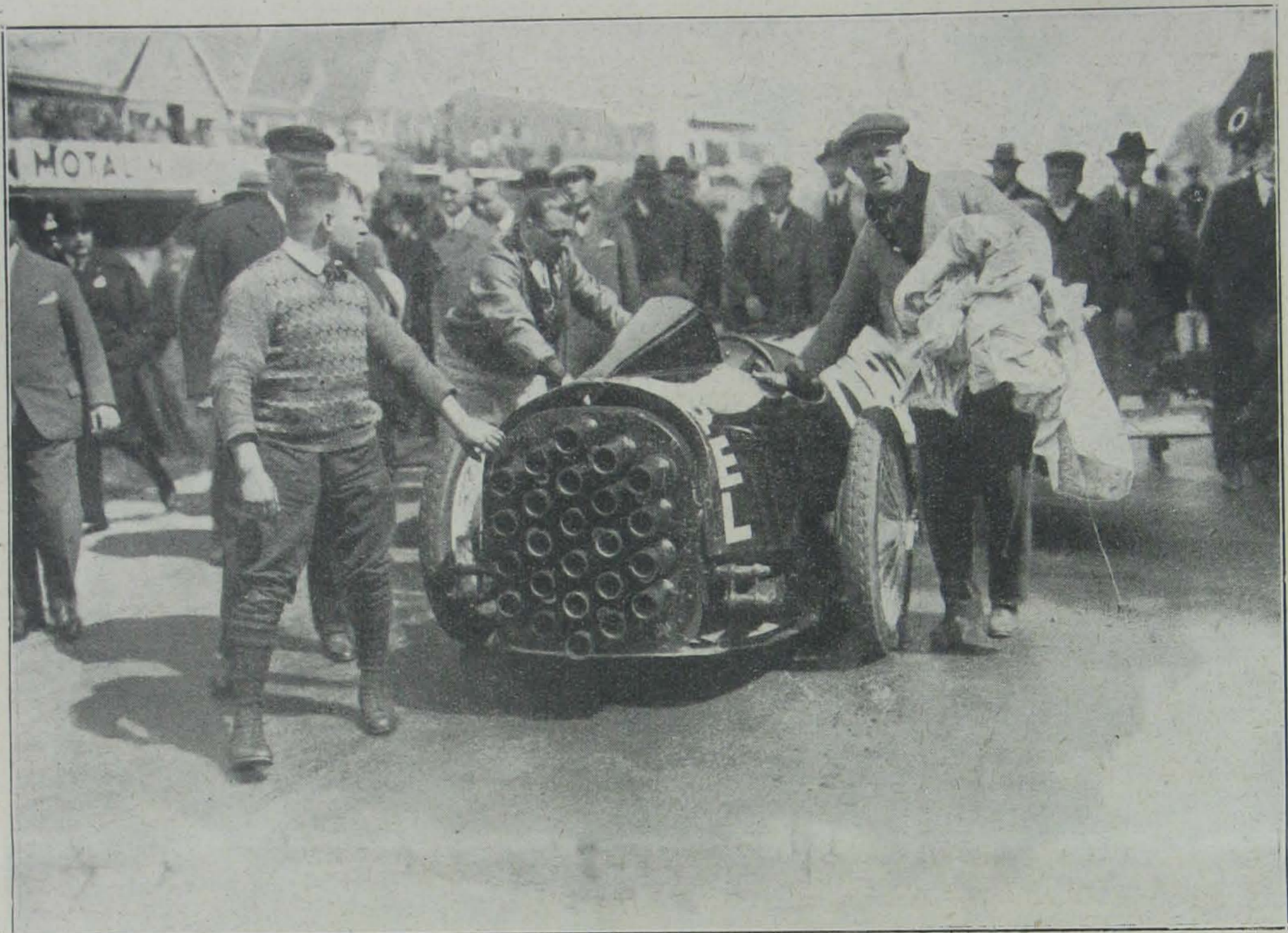
Fritz von Opel rakétaautójával a berlini Avus pályán starthoz áll. A rakétaautó hátsó részében látjuk a kipuffogókat, ahova a rakéták kerülnek.
