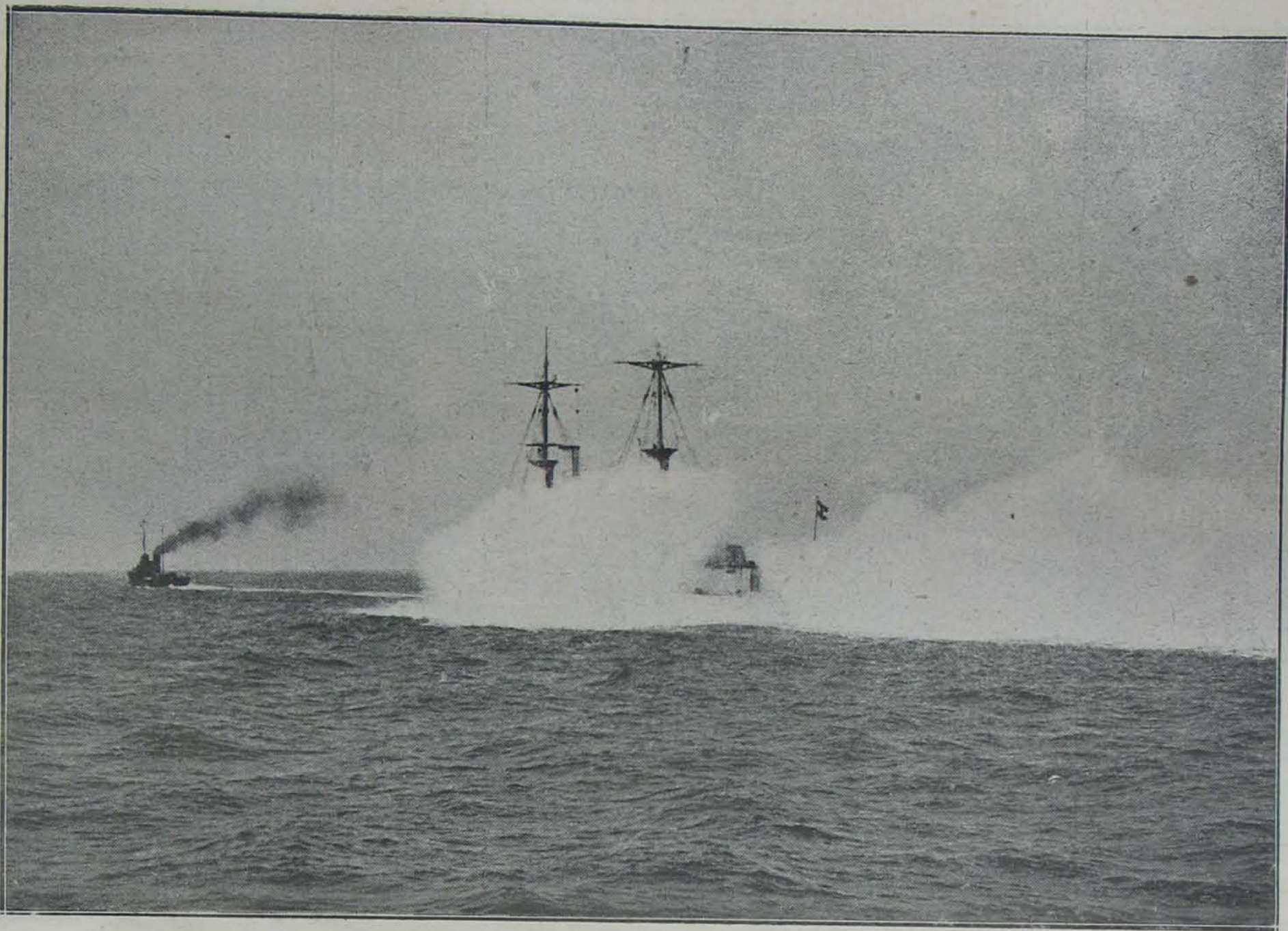
A „Zähringen” német páncélos cirkáló, a kísérteties hajó, amelyen senki sem tartózkodik s ennek ellenére is ép úgy manőverez s minden tekintetben úgy működik, mintha kezelő személyzet volna rajta. A képen látható „Blitz” nevű torpedórombolóról irányítják rádió útján, amivel ködfelhőbe is lehet burkolni a cirkálót.
