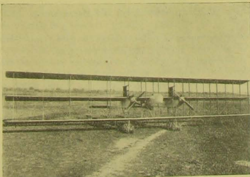
3. ábra: Háromsíkú, vékonyszárnyú, kétmotoros repülőgép (szárazföldi) futószerkezettel és 2 kétszárnyú húzó légcsonnyal.
