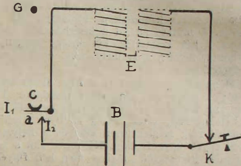
A „személyi hibát” kimutató készülék vázlatos rajza. K = rugós áramkapcsoló; B = galvánelemek; C = csésze; G = golyó; E = elektromágnesek. Az E elektromágnesen átvett áramkör I_1 és I_2 kontaktus-végek között a = 0.1 mm. hézaggal van megszakítva.
