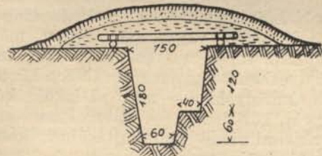
5. sz. ábra. Gázbiztossá tehető szilárdbiztos óvóhelyárok.
