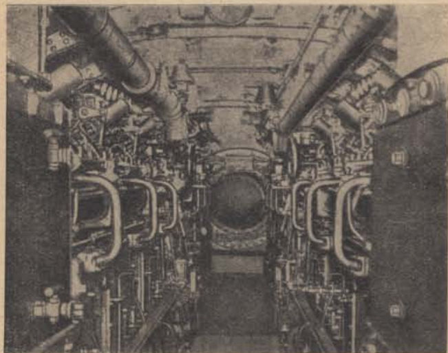
Búvárnaszád Diesel-motorjainak a helyisége. Középen a háttérben látszó kerek ajtó vízhatlanul elzárható. Ilyen ajtók (Schotten) választják el egymástól a naszád összes helyiségeit.
