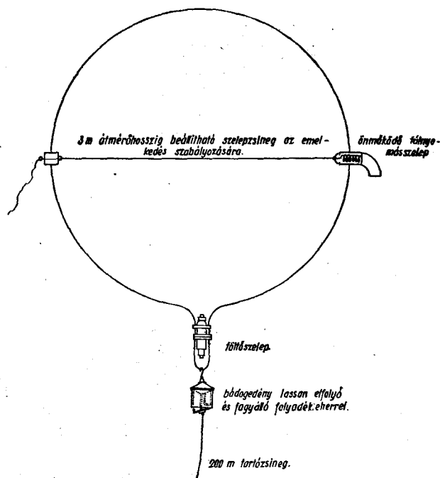
A romboló-ballon szerkezete.
