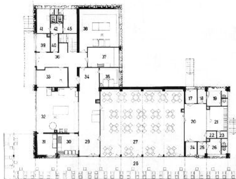
Földszint alaprajz: KOŠEK
