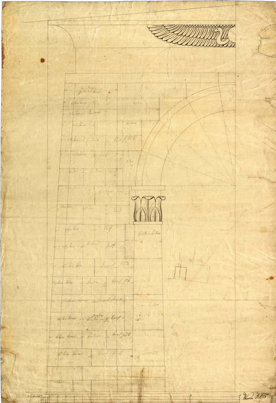
2. kép: A Sötétkapu déli homlokzatának kőkiosztási terve (PL TGy 60. [Rj. 58. P. 58.])
