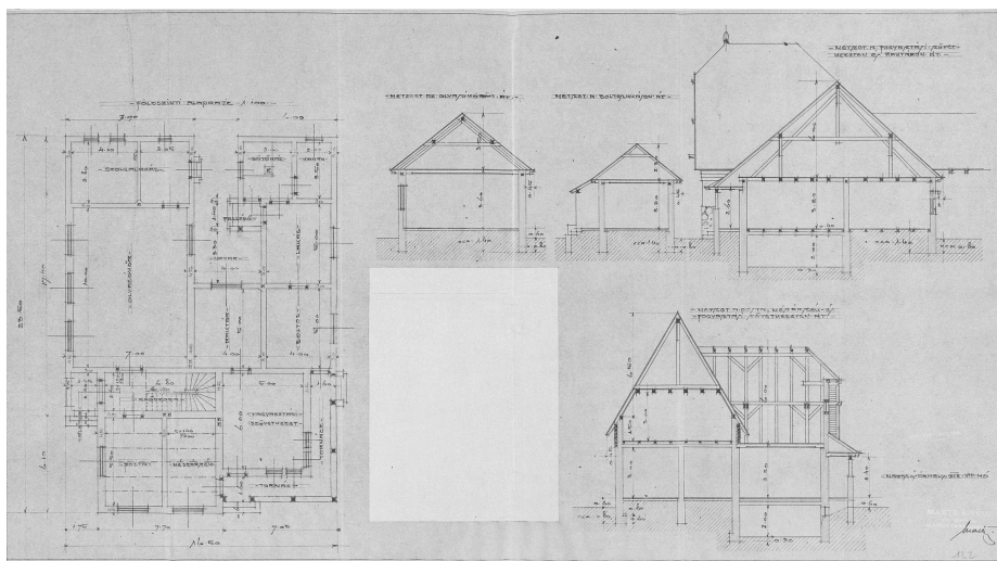
2. kép: Marosfelfalui népház (Maros-Torda megye) tervdarja
