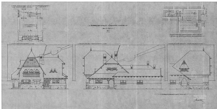
1. kép: Marosfelfalui népház (Maros-Torda megye) tervrajza
