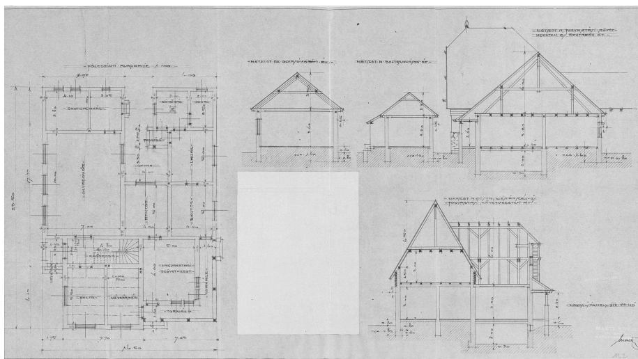
2. kép: Marosfelfalui népház (Maros-Torda megye) tervrajza
