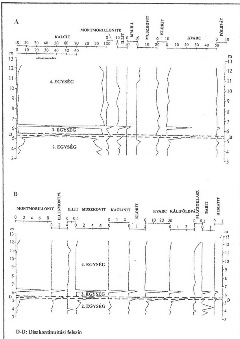
4. ábra: A Vár-hegy édesvízi mészkővének ásványos összetétele, A és B) az édesvízi mészkő típusszelvényének ásványos összetétele a röntgendifrakciós vizsgálatok alapján, A) teljes kőzetminta, B) oldási maradék, C, D, E és F) az édesvízmészkő típusszelvényének jellemző termoanalitikai (TG és DTG) görbéi, C) a laminált édesvízi mészkő (2. egység) oldási maradéka, D) a paleotalaj (3. egység) "B" szintje, E) a paleotalaj (3. egység) "A" szintje, F) a tömeges édesvízi mészkő (4. egység) oldási maradéka, G) a 2. és 4. egység kalcitjának korrigált bomlási hőmérséklete (100 mg kalcitra számolva, szórással) Fig. 4 Mineralogy of Vár-hegy travertine A and B) XRD mineralogical logs of travertine key-section: A) whole sample, B) insoluble residue, C, D, E and F) typical thermoanalytical (TG and DTG) curves of travertine key-section: C) insoluble residue of laminated travertine /Unit 2/, D) palaeosoil, "B" horizon /Unit 3/, E) palaeosoil, "A" horizon /Unit 3/, F) insoluble residue of massive travertine /Unit 4/, G) decomposition temperature ( T_{corr} ) recalculated to 100 mgs of calcite in Unit 2 and Unit 4 with dispersion
