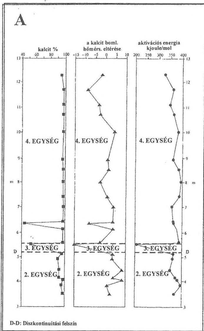
5. ábra: A kalcit tartalom eltérése, valamint a kalcit bomlási hőmérsékletének aktivációs energiája és a \delta^{18}\text{O} eloszlás korrelációja a Vár-hegy édesvízi mészkövének szelvényében A) a korrigált bomlási hőmérsékletéhez tartozó kalcit tartalom eltérés és a kalcit bomlás aktivációs energiájának kapcsolata a TA mérések alapján (100 mg kalcitra számolva) B) a \delta^{18}\text{O} eloszlás és a korrigált bomlási hőmérséklet kapcsolata. Fig. 5 Calcite content deviation, activation energy of calcite decomposition temperature and correlation to \delta^{18}\text{O} of Vár-hegy travertine. A) calcite content deviation of corrected decomposition temperature (recalculated to 100 mgs of calcite) and activation energy of calcite decomposition measured by TA, B) correlation between corrected decomposition temperature and \delta^{18}\text{O}
