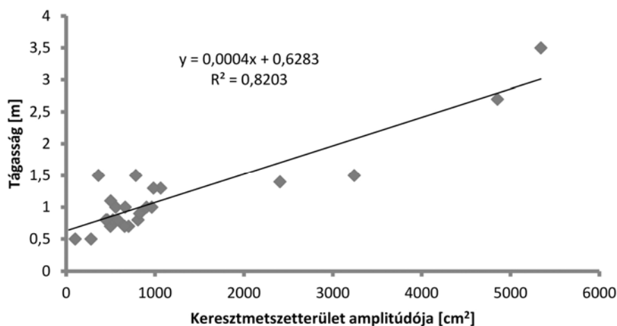
7. ábra: A különböző vályúrendszerek fővályúinak fő- és B típusú mellékvályúin a maximum helyek amplitúdója és tágassága közti kapcsolat
