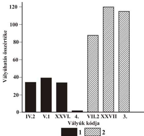
8. ábra: Különböző maximum gyakoriságú fővályúkra számított vályúhatás összértékek
