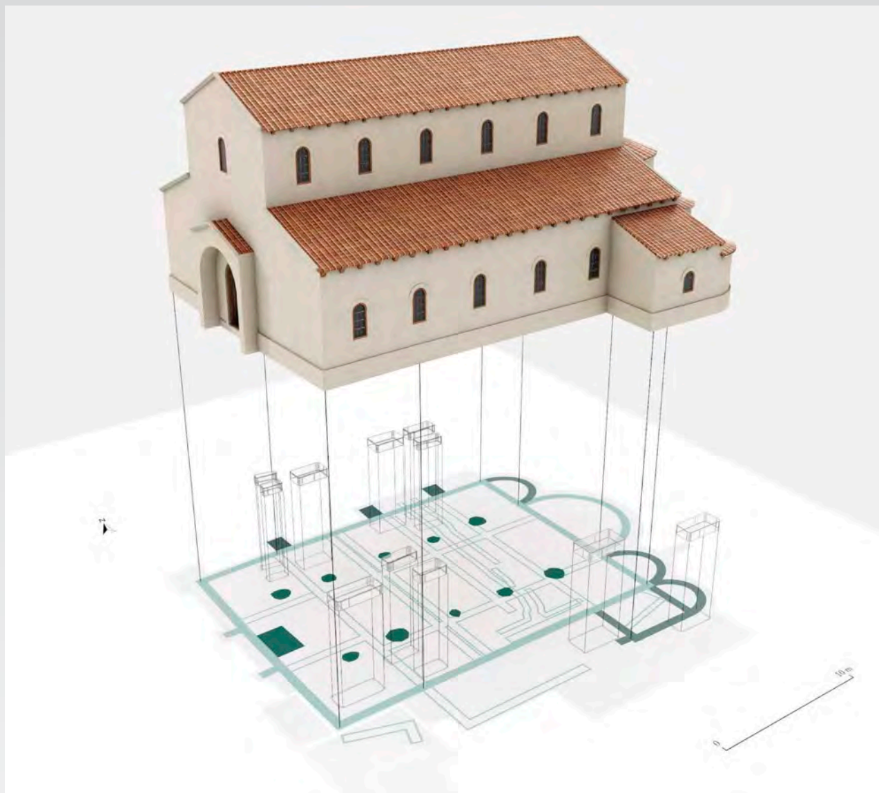
A bazilika alaprajza és épületének rekonstrukciója (készítette: Narmer Építészeti Stúdió, Vasáros Zsolt, Kiss Gábor és Heinrich-Tamácska Orsolya)
