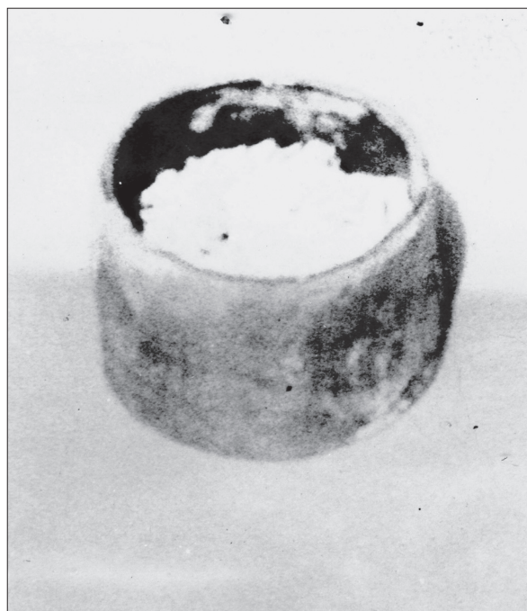
5. ábra Mérték. Szájátmérője 4,6 cm, magassága 3,6 cm, talpátmérője 5,2 cm. Szaruból készült, az alja fából van becsinálva. Mázból 7 megy egy kilóba, ha darabosabb, akkor nyolc. A mérték szerint vannak a máz és festék összetételek megadva
