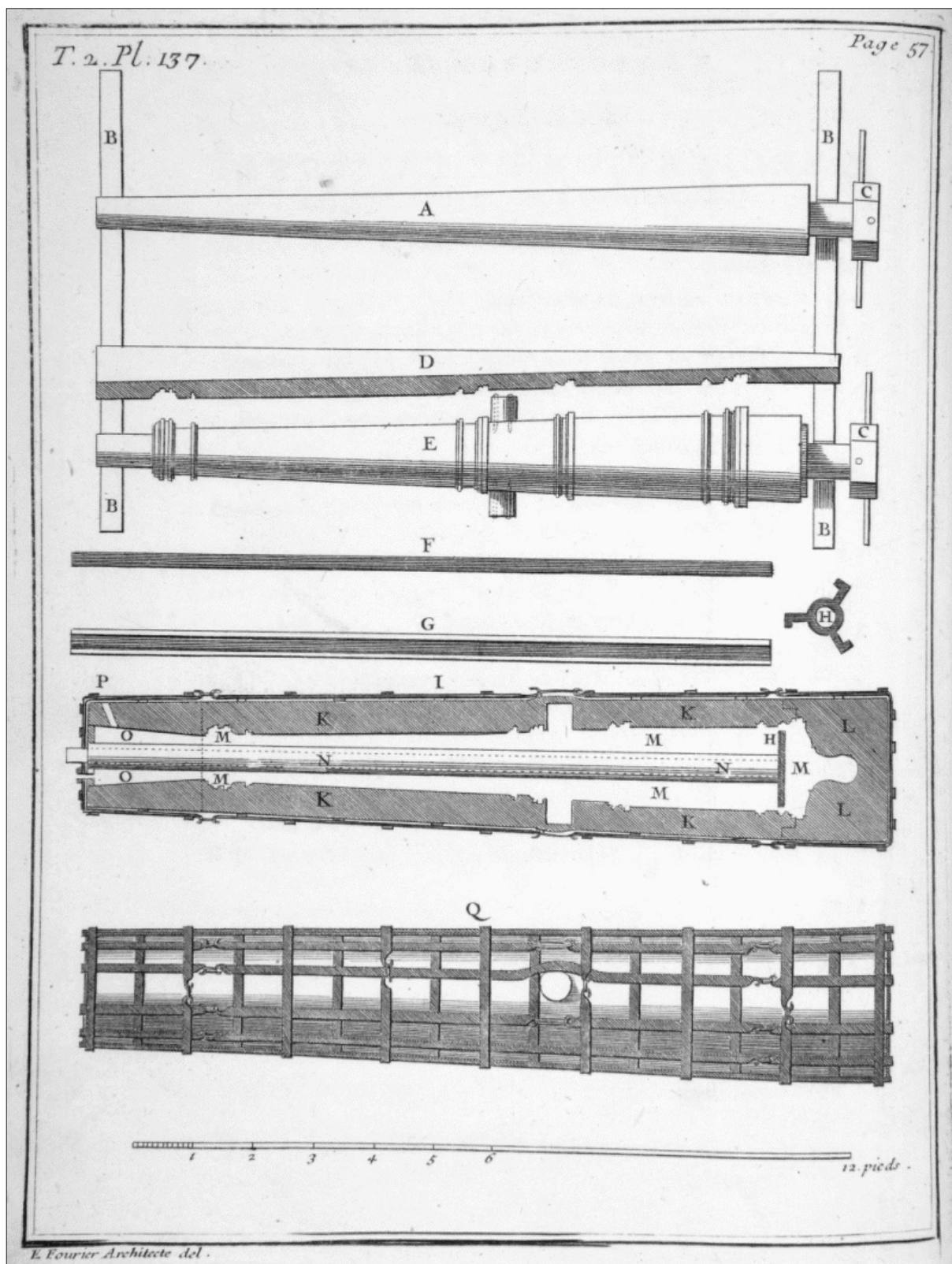
1. ábra Az öntőminta és az öntőforma elkészítésének lépései. (Surirey de Saint Remy, Pierre: Memoires d'Artillerie , Párizs, 1707.) A. Pózna; B. Bak; C. Kézikerék forgatáshoz; D. Sablon; E. Kész minta; F. A mag hordozója (keményfa vagy kovácsvas); G. A mag agyagköpenye; H. Magtámasz; I. Az öntőforma vasalása; K. Az öntőforma fő része; L. A csőfar öntőformája; M. Az ágyúcsövet kialakító formaüreg; N. Az ágyú furatát kialakító mag; O. A tápfejet kialakító formaüreg; P. A tápfejet kialakító formarész (itt külön elkészítve) ; Q. A kész öntőforma
