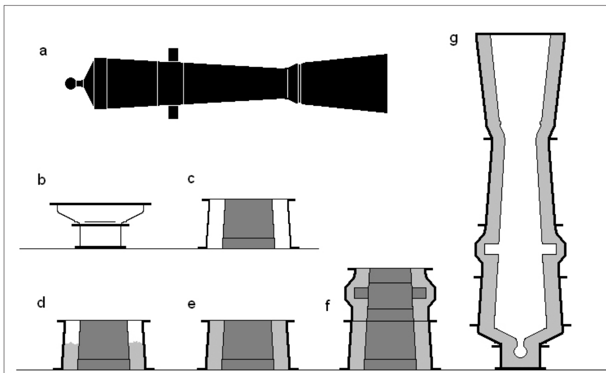
4. ábra Ágyú formázása formaszekrényvel öntőhomokba.
