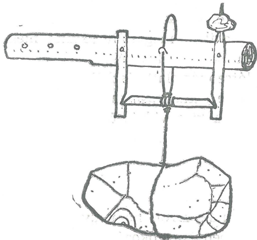
Nyestfogó hurok, kővel nehezített dróthurok (faág csontjára szegzik).
