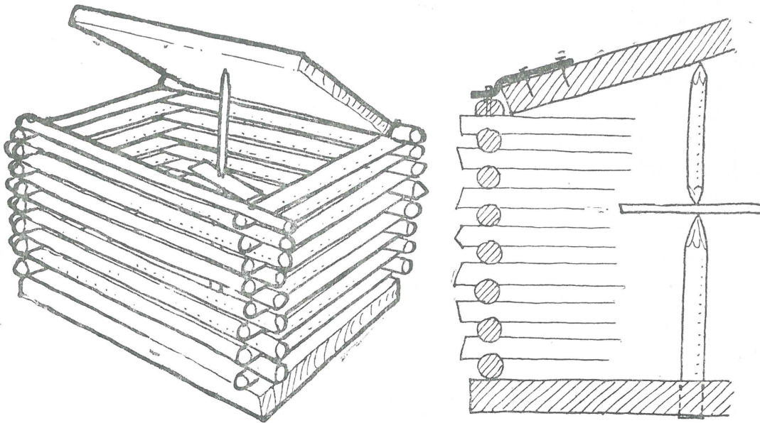
Verébfogó galicka és szerkezeti rajza.
