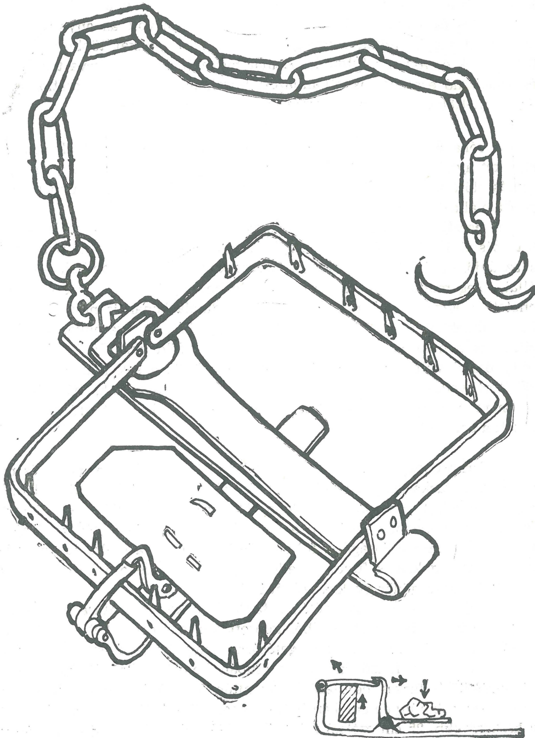
Vaskaptány láncra szerelt horoggal medvefogáshoz (lent: kioldószerkezete).
