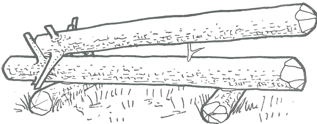
Nyestüttető, kezdetleges (két egymásra fektetett gerenda).
