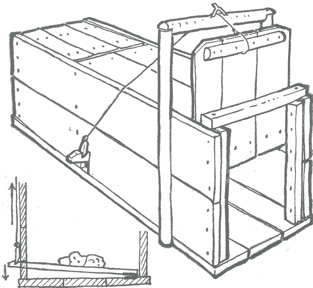
Rókaláda (h : 150 cm, sz. : 55 cm) és kioldószerkezete.
