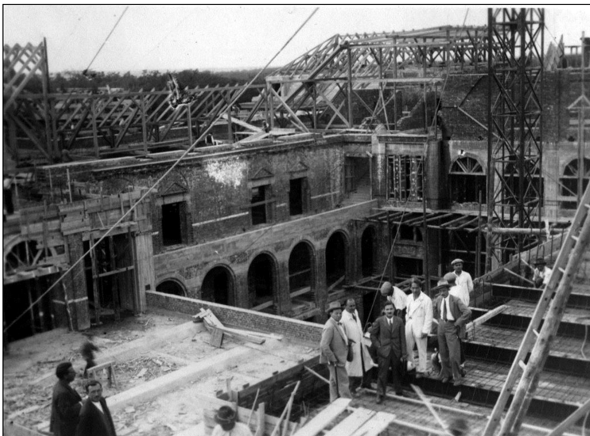
2. kép A Debreceni Egyetem Központi épülete kivitelezés közben I. 8
