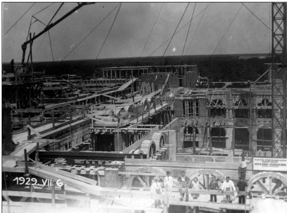
3. kép A Debreceni Egyetem Központi épülete kivitelezés közben II. 9
