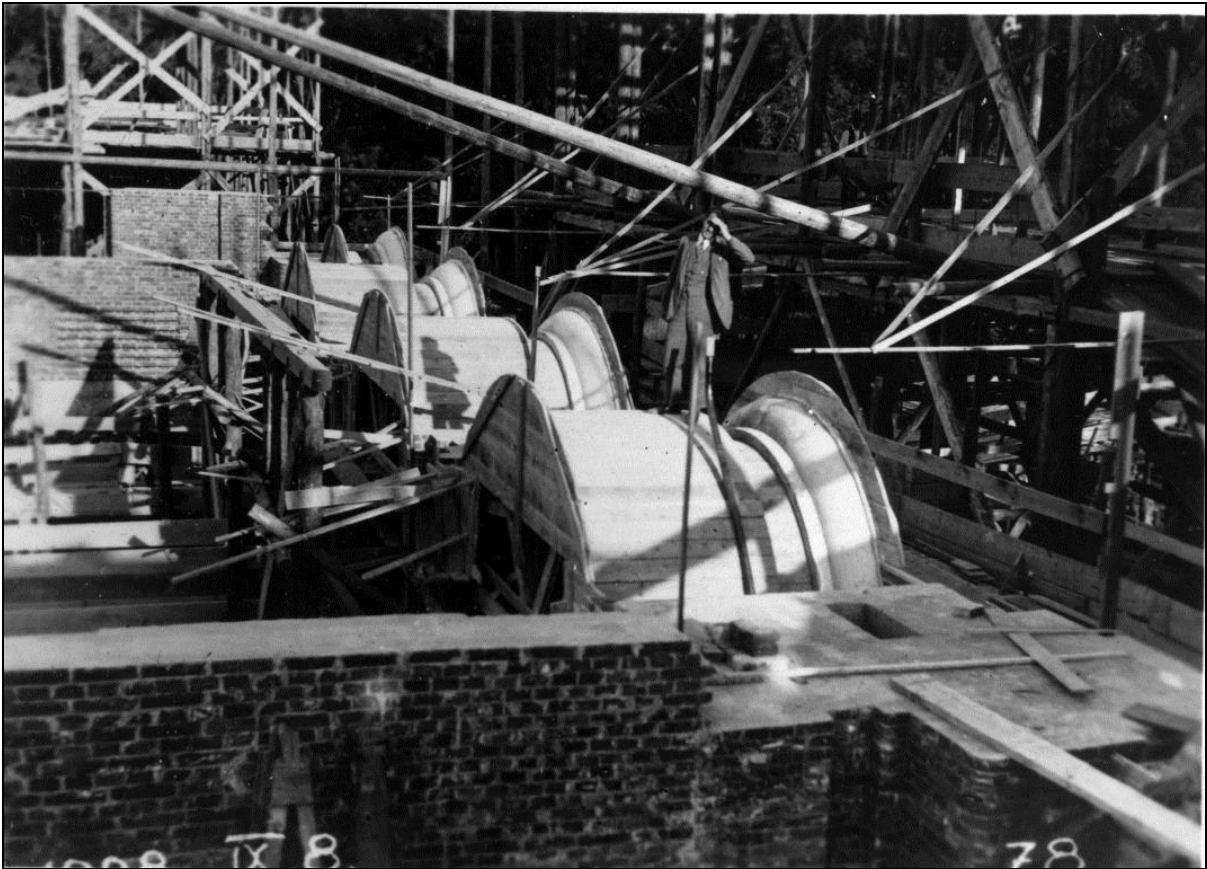
4. kép A Debreceni Egyetem Központi épülete kivitelezés közben III. 10
