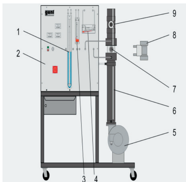
4. ábra HM-210 Radiális ventilátor mérőállomás „U” csöves manométer 2. Alap panel, 3. Venturi-cső nyomásmérő 4. Ferde csöves manométer 5. Radiális ventilátor 6. nyomócső 7. Szabályzó 8. Venturi-cső
