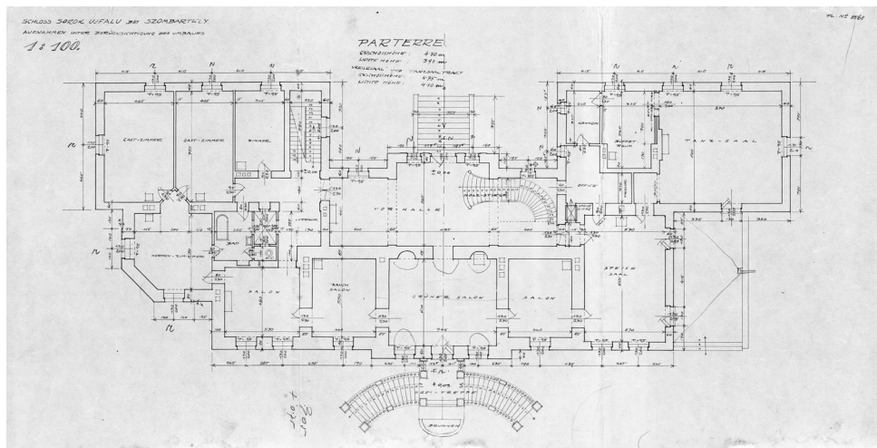
A sorokújfalui kastély földszinti alaprajza, 1927 MNL VaML Sz hely. ép. váll. ir. 33. doboz. Sorokújfalu, 1927–1930.
