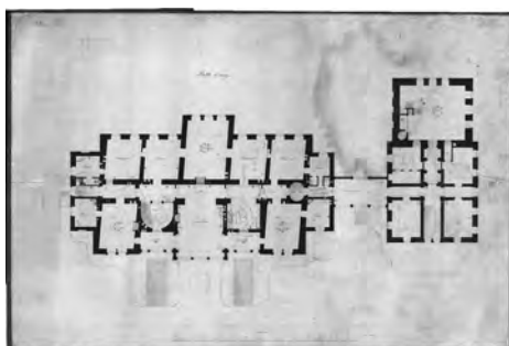
6. kép: A kastély főépületének első emeleti és melléképületének földszinti alaprajza, 2. sz. kiviteli tervsorozat, 1846.
