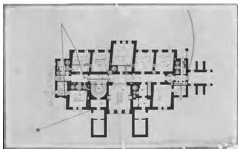
1. kép: A kastély főépületének földszinti alaprajza, 1. sz. kiviteli tervsorozat, 1846. Szombathely, Magyar Nemzeti Levéltár, Vas Megyei Levéltár
