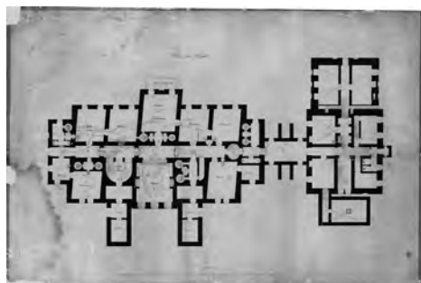
5. kép: A kastély főépületének földszinti és melléképületének pincszinti alaprajza, 2. sz. kiviteli tervsorozat, 1846.
