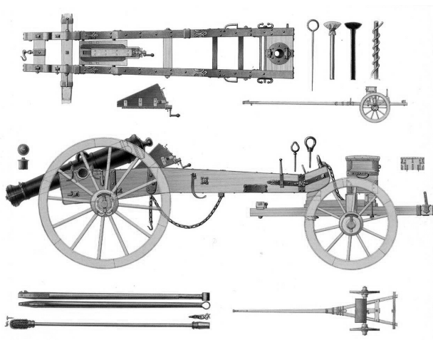
Hatfontos ágyú rajza
