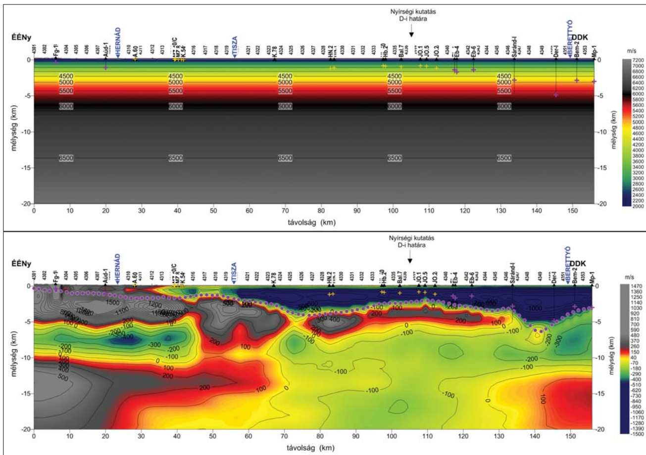
19. ábra Átlagos sebességtrend (felül) és a sebességanomália (alul), azaz az átlagos sebességmenettől való eltérés a CEL04-szelvény mentén (lila pöttyökkel a Kilényi–Sefara-féle medencealjzat-mélység van jelölve)
