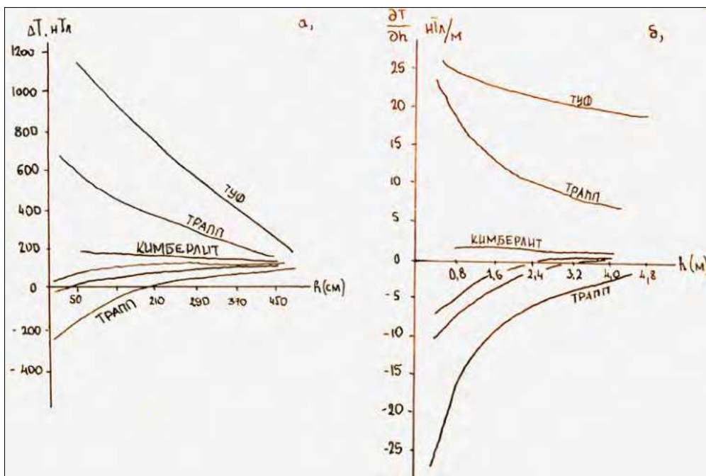
13. ábra | A mágnesesanomália-tér ( \Delta T ) és a mágneses vertikális gradiens ( \Delta T'_z ) változása a mérési magasság függvényében. A trappbazaltok változatosságát (megíratlan görbékkel) a remanens mágnesezettség okozza. (Nyikulin 1982 alapján, Kiss 1986 – ТУФ = tufa, ТРАПП = trappbazalt, КИМБЕРЛИТ = kimberlit)
