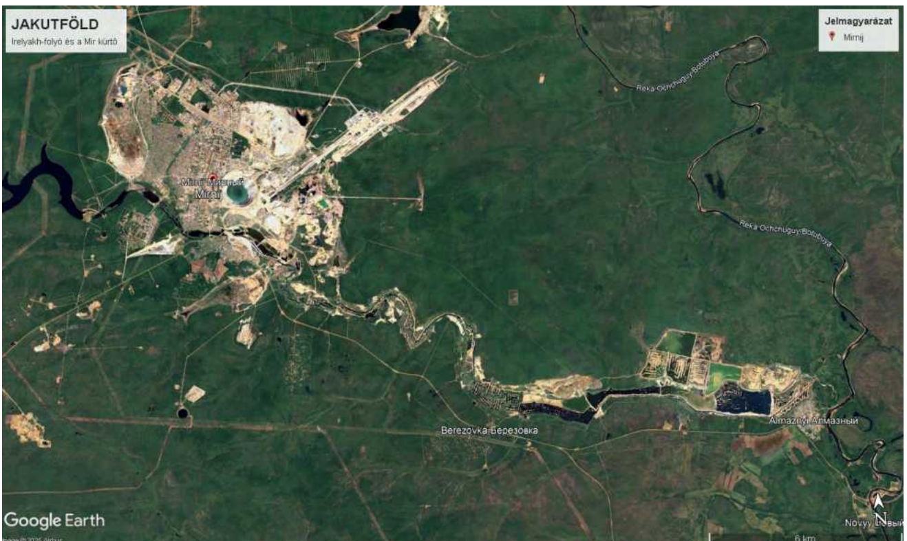
3. ábra | A kibányászott Mír kimberlitkürtő a Google Earth felületén is azonosítható (balra Mírnij település benne a Mír kimberlitkürtő, jobbra az Irel'yakh folyó 6) menti torlatkitermelés nyomai az Almaznij (magyarul Gyémántos) nevű településsel) Figure 3 | The mined Mir kimberlite pipe can also be identified on Google Earth (on the left is the town of Mírnij, inside the Mír kimberlite pipe, and on the right are traces of tailings mining along the Irel'yakh River, with the town of Almaznij, meaning “Diamond”)
