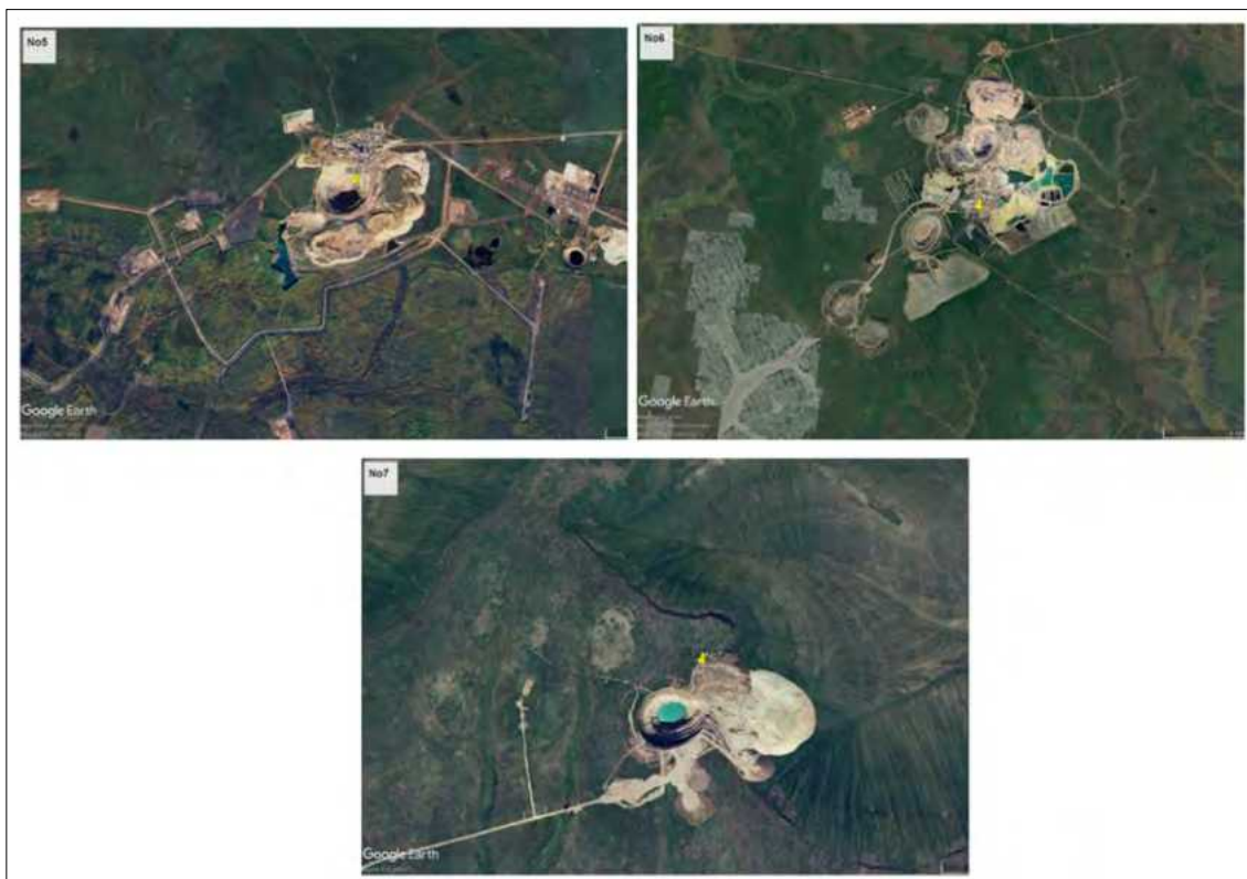
28. ábra Kimberlitkürtők a Google Earth felvételeken: No1 – Ismeretlen nevű; No2 – Udacsnaja, Polarnaja, Zarnyica; No3 – Ajhal No4 – Mír; No5 – Internacionalnaja; No6 – Ismeretlen nevű; No7 – Szütükanszkaja
