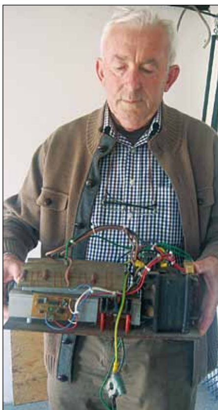
Íme, egy elkobzott, a hal kábítására, házi-lag összerakott elektromos berendezés
