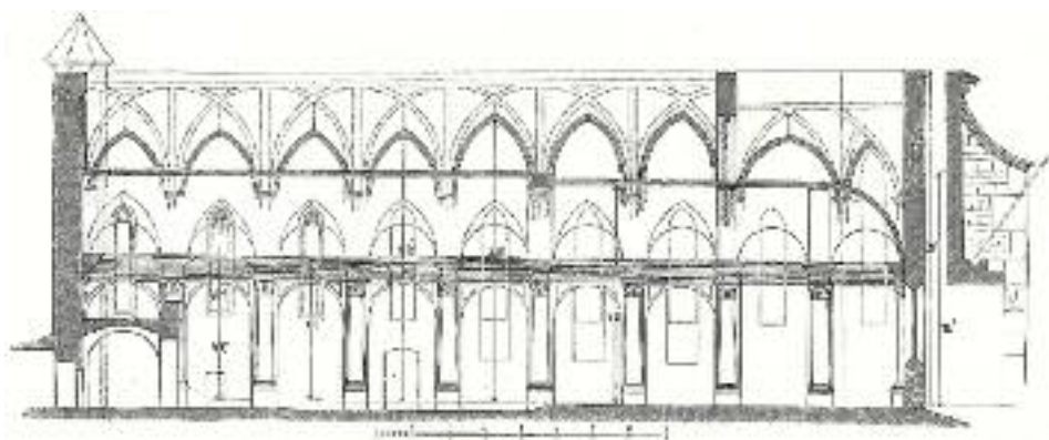
4. kép Stornó Ferenc felmérte hosszmetset és rekonstrukció, 1880
