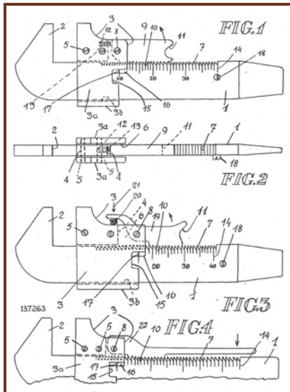
Az egyik általa tervezett, állítható csavarkulcs szabadalmi rajza
