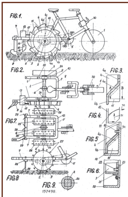
Láb- vagy motorhajtásos, talajaprító-, szántó-, vető- és talajlazító gép terve
