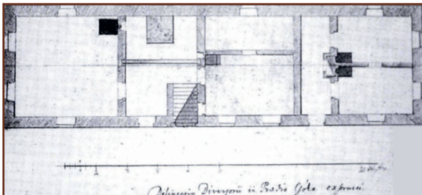
A Csókai csárda alaprajza
