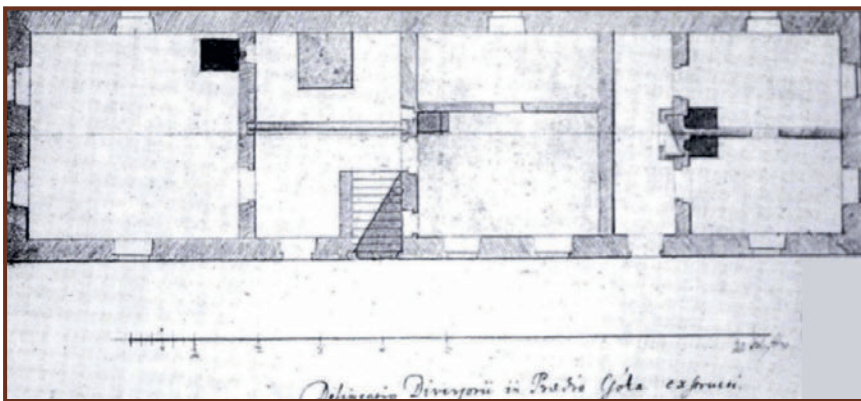
A Csókai csárda alaprajza
