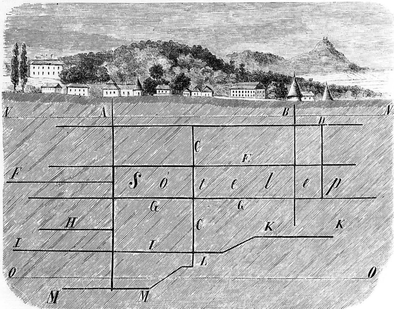
A wielieskai sóbánya átmetszete. (Rajz. Myskovszky V. Szövege a 22. lapon.)
