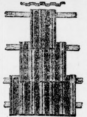
Zombolyai gyártmány. Szab. biztonsági preselt átfedőcserep 253. sz.
