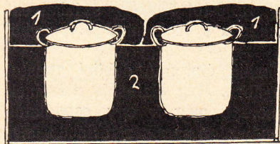
Kétedényes főzőláda keresztmetszete. 1. Párnák. 2. Fagyapót.
